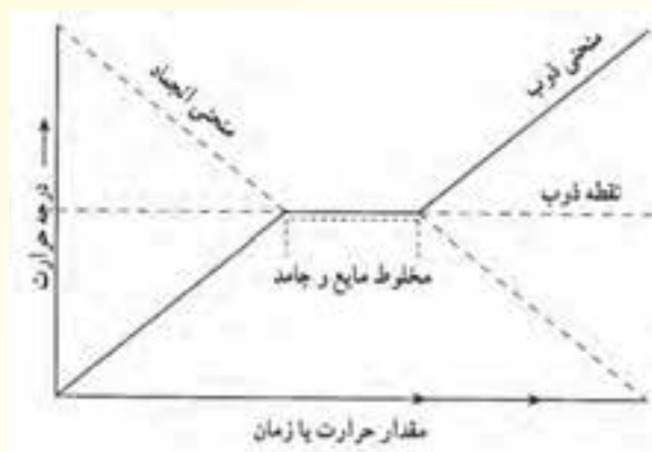
شکل ۱-۴- منحنی ذوب و انجماد فلز خالص
