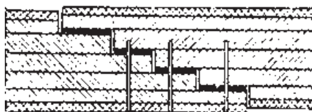
شکل ۱۱-۱۲- اتصال قطعات نوار به وسیله ولکانیزاسیون [۳۸]
