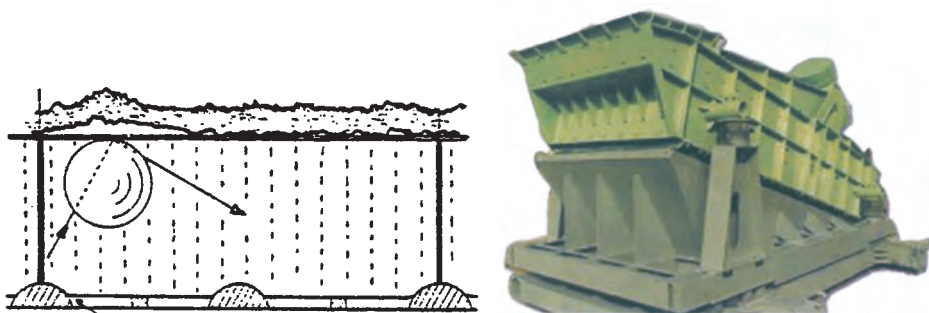
غربال برای بار مرطوب
