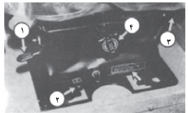
شکل ۱۷-۵- تنظیم صندلی راننده
