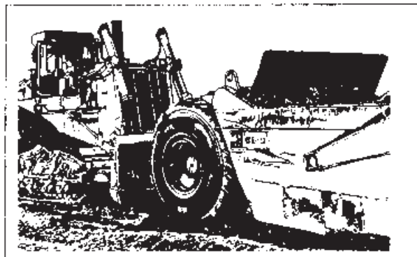
شکل ۵-۵۹ - هل دادن اسکرپر توسط بولدوزر سرعت حرکت بولدوزر نباید بیش از ۵ کیلومتر در ساعت، سریع تر از حرکت اسکرپر باشد.
