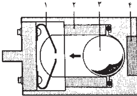
شکل ۲۲-۲ - سنسور الکترومکانیکی
