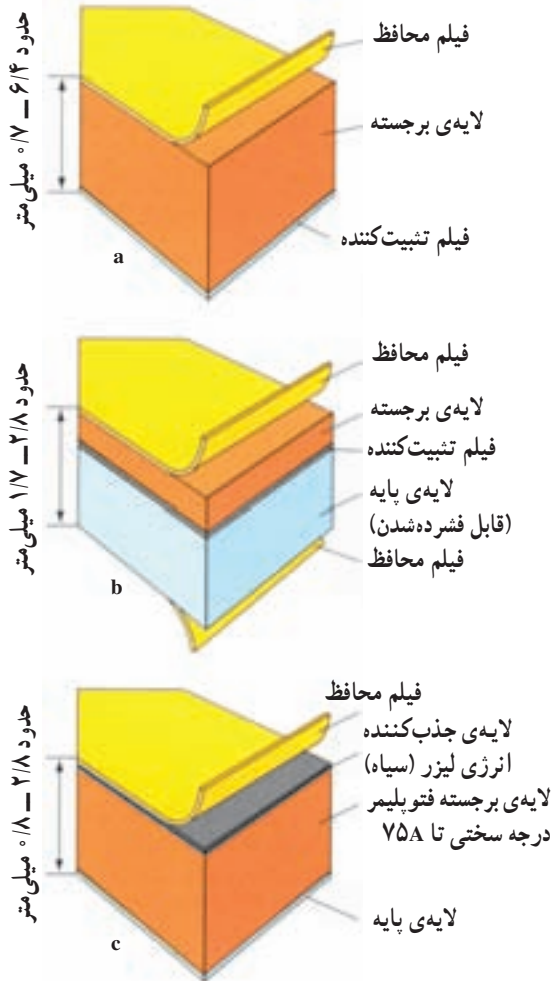
شکل ۳-۴ ساختمان تعدادی از پلیت‌های فلکسوگرافی: پلیت a — تک لایه (BASF)، پلیت b — چند لایه (BASF)، پلیت c — برای سیستم کامپیوتر به پلیت (digiflex, BASF)
