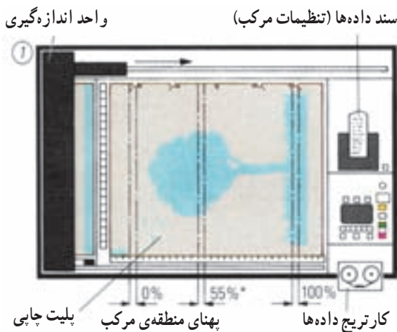
شکل ۶-۲۸— اسکن منطقه به منطقه پلیت چاپی و امکان ضبط داده ها
