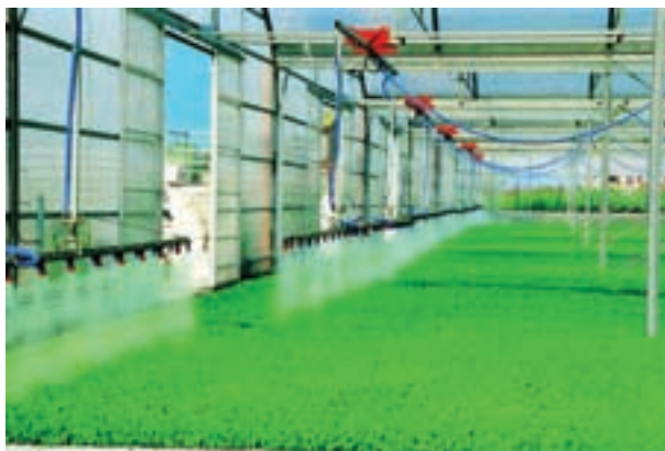
شکل ۹۹-۷- آبیاری مه‌پاشی در گلخانه
