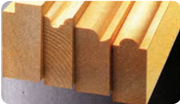
شکل ۴-۴ چند نمونه لبه‌چسبان چوبی ابزار خورده
