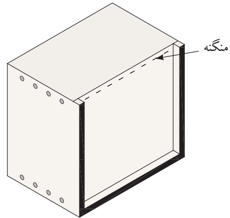
شكل ۶-۱۹ پشت بند به سقف منگنه مى شود.
