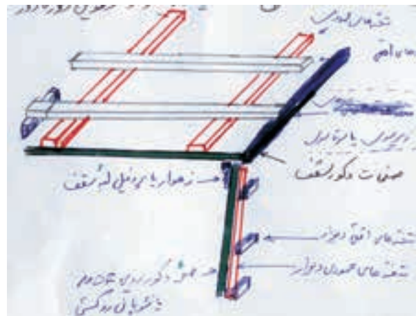
شکل ۷-۴۳ استفاده از L یا گونیای ۹۰ درجه برای چسباندن چوب‌های شیب‌دار
