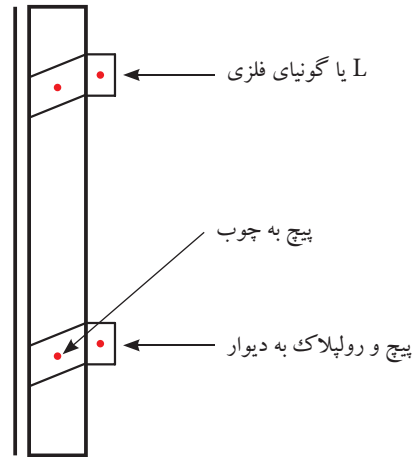
شکل ۲۲-۷ استفاده از L یا گونیا فلزی ۹۰ درجه برای چسباندن چوب‌های شیب‌دار
