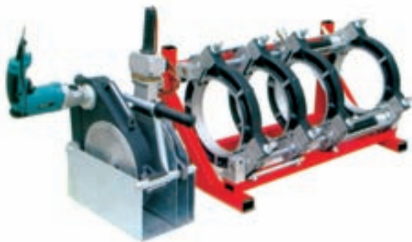
شکل ۲-۳۶- دستگاه جوش
