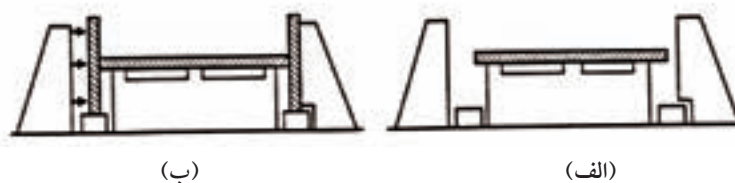
شکل ۱۱-۶- مونتاز تیرورق در قالب
