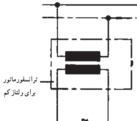
شکل ۱۰-۱- ترانس کاهنده ولتاژ
