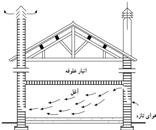
شکل ۳۰-۳ - سیستم مختلط تهویه
