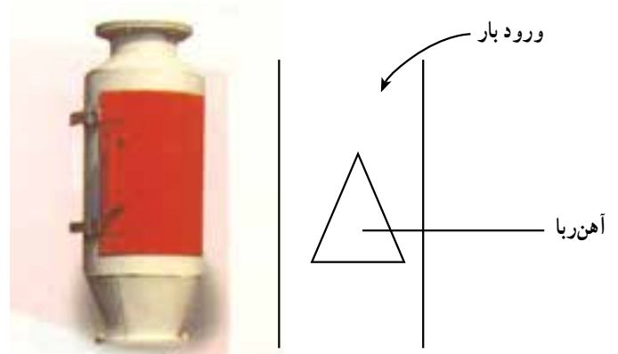
شکل ۹-۱- شمای آهن‌گیر
