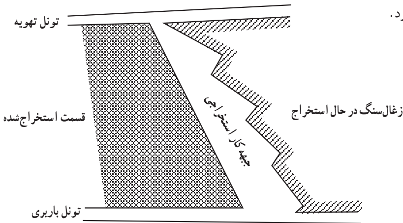
شکل ۸-۹- روش استخراج جبهه کار دندانۀ اره‌ای
