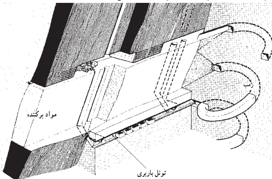
شکل ۱۰-۷- روش استخراج کندن و آکندن
