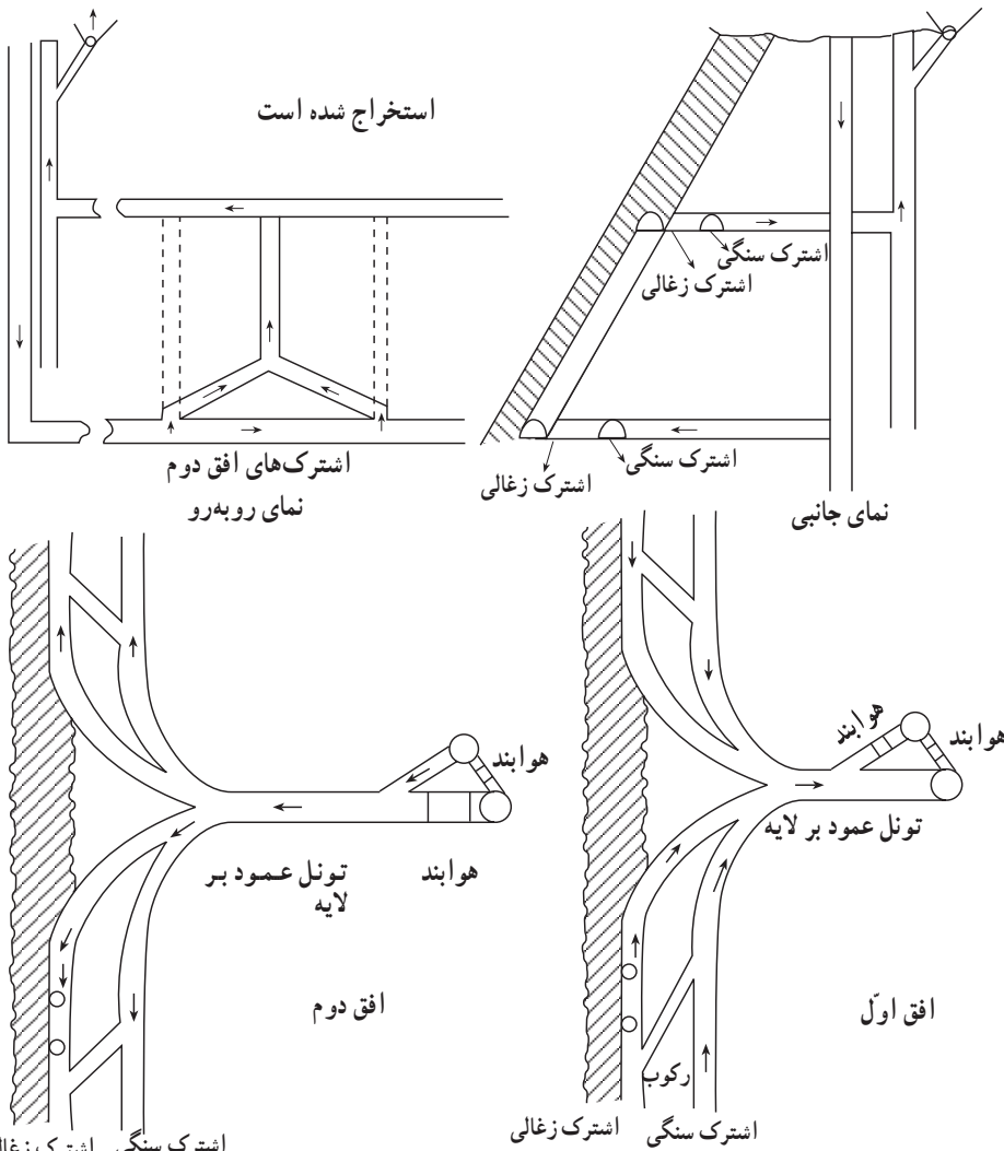
اشترک سنگی اشترک زغالی نمای از بالا افق اول
