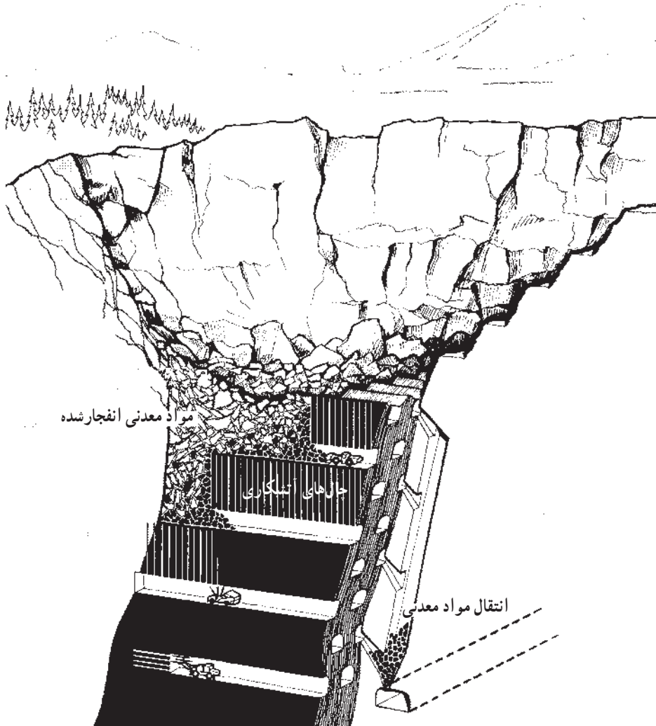
شکل ۱۶-۷- روش استخراج تخریب در طبقات فرعی
