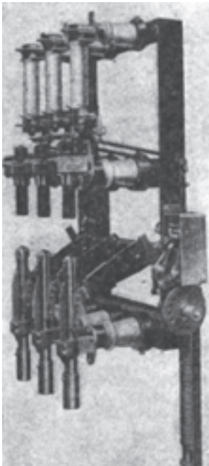
شکل ۸-۱۵- یک سکسیونر قابل قطع زیر بار با محفظه‌ی احتراق
