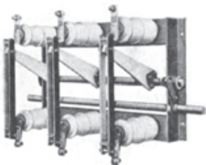
شکل ۸-۱۳ - سکسیونر کشویی
