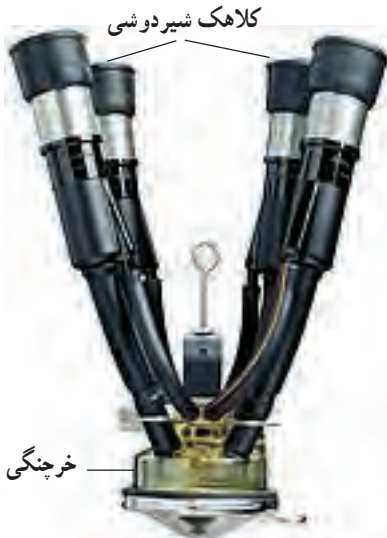
شکل ۴۴-۴- خوشه شیردوش
