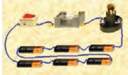
شکل ۱-۵۴ مدار لامپ با ۶ پیل ۱/۵ ولتی
