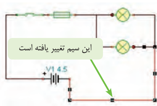
شکل ۱-۵۳ اصلاح نقشه‌ی فنی مدار از طریق جابه‌جایی خطوط و قطعات
