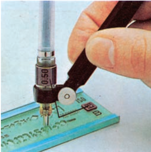
شکل ۲۸-۱- شابلون حروف و اعداد
