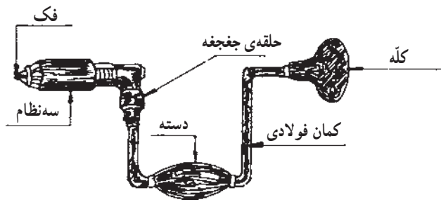
شکل ۱-۳۱- دریل دستی جفجه‌ای
