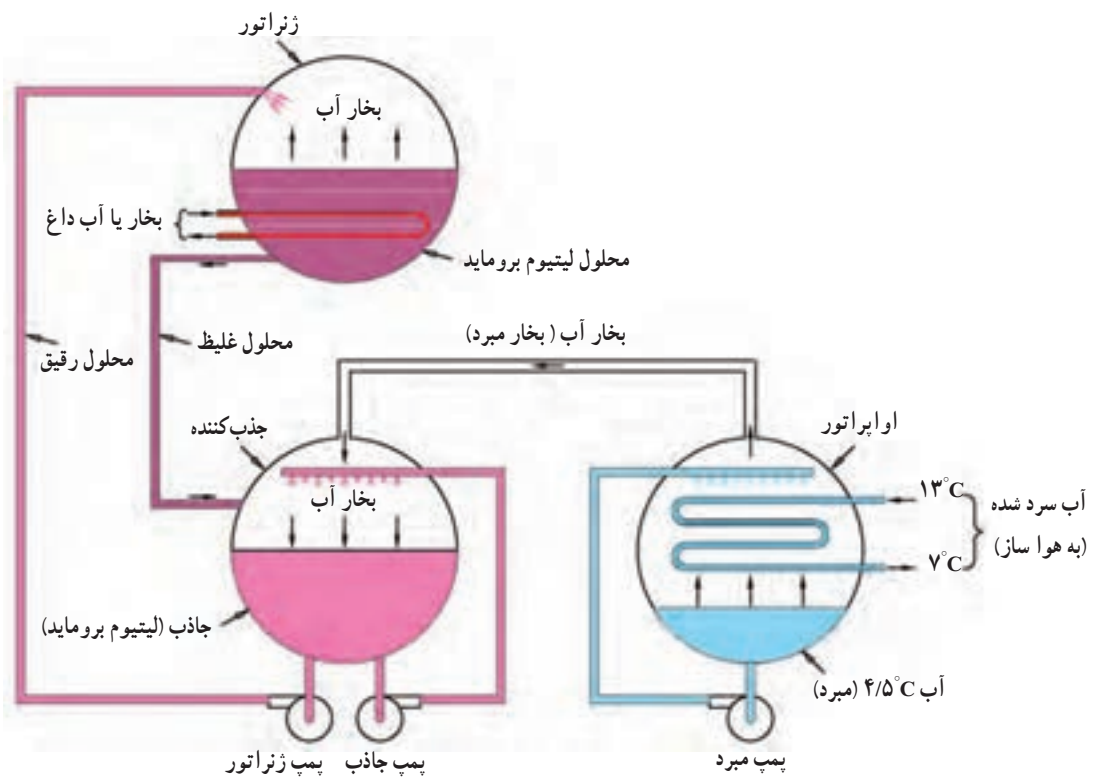
شکل ۳-۱۲- برای رفع مشکل اول به سیستم یک زراتور اضافه می کنیم.
