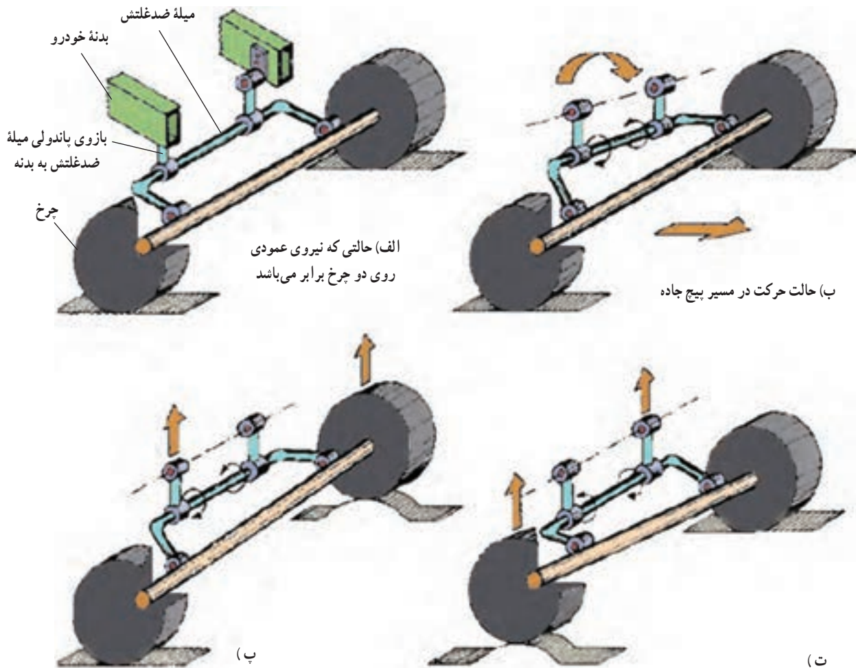
شکل ۲۷-۷- میله ضد غلتش و نحوه عملکرد آن در حالت های مختلف
