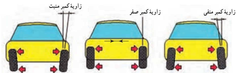
شکل ۱۰-۷- حالات‌های مختلف زاویه کمبر چرخ
