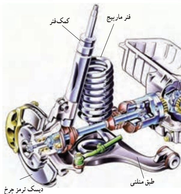
شکل ۳۶-۷- مکانیزم تعلیق استرات دمپر
