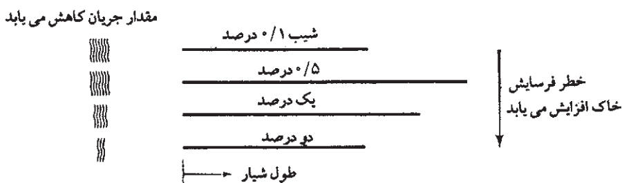
شکل ۸-۹- عوامل مؤثر در تعیین طول شیار
