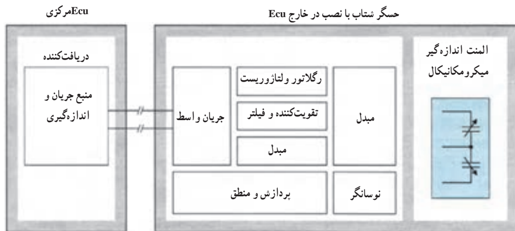
شکل ۳-۵-۳ ASIC واسطه برای ارزیابی سیگنال حسگر شتاب (یک پارچه با Ecu)
