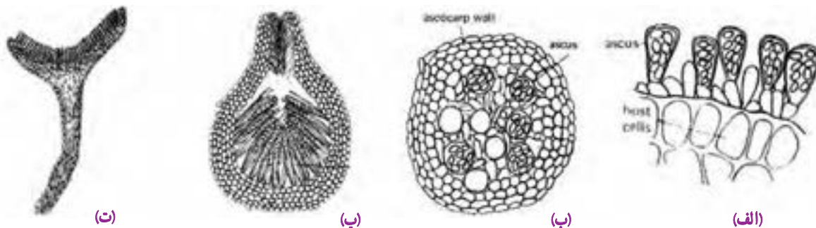
الف) زیموتشیوم (ب) کلیستوتشیوم (ب) پری تشیوم (ت) آپوتشیوم شکل ۴-۴ رده بندی آسکومایکوتینا بر اساس نوع آسکوکارپ
