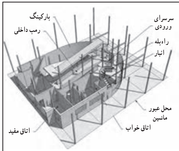
استفاده از پلان آزاد در ویلا ساوی توسط لوکوربوزیه، دیوارها نقش جداکننده دارند و سهمی از انتقال بار ندارند.
