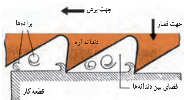
شکل ۱-۱- دندانه‌ی تیغه‌اره
