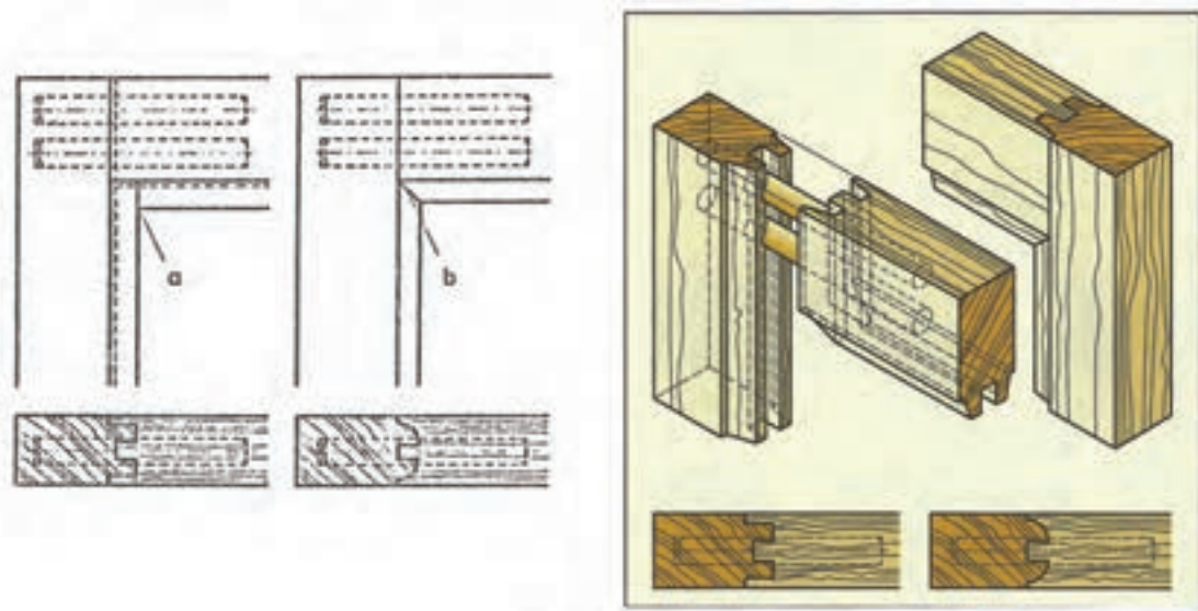
شکل ۵-۶۵: ترسیم اتصال گوشه‌ای دوبر با پروفیل دو طرفه (درز گوشه‌ قاب فارسی و گونیایی) در دو نمای رو به رو و بالا و تصویر مجسم اتصال و تصویر مجسم انفجاری
