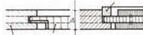
شکل (۵-۱۱۵) ترسیم اتصال قاب و تنکه هشت نوع مختلف صفحه‌چوبی تنکه از صفحات چندلایي با تنکه دوراهه شده با پوشش فلزی و قاب چوبی
