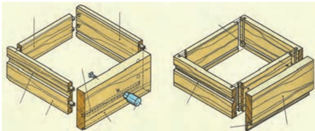
شکل (۵-۴۶) تصویر مجسم انفجاری جعبه با اتصالات گوشه‌ای
