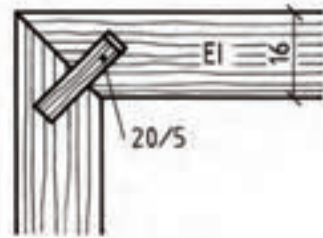
شکل (۵-۷۸) نقشه برش مصنوعی با زاویه ۴۵ درجه
