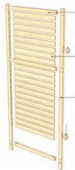
شکل (۵-۳۰) تصویر مجسم پارتیشن نوع دیگر، با قیدهای کرکره مانند و اتصالات گوشه‌ای فاق و زبانه و اتصال میانی فاق و زبانه و کم و زبانه.
