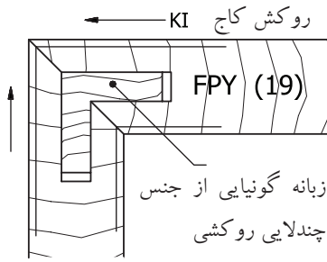
شکل (۵-۱۱۲) ترسیم اتصال صفحه‌ای گوشه‌فارسی با دوپل گونیايي از جنس چندلایي روکشی
