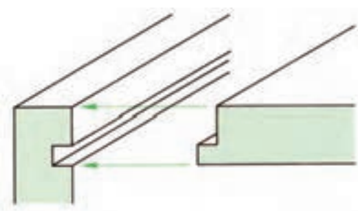
شکل (۵-۷۵) تصویر مجسم انفجاری قلیف زبانه سرخود
