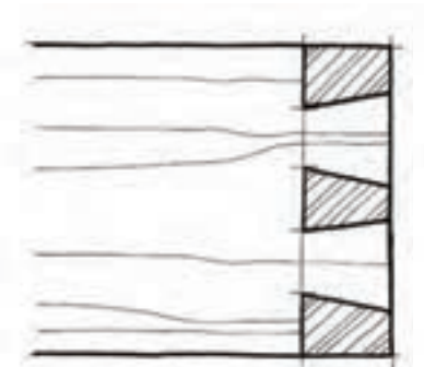
شکل (۵-۱۰۷) ترسیم اتصال دم چلچله ساده دو زبانه ۱:۱ M
