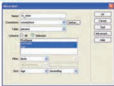
شکل ۲۰-۱۰ ایجاد Recordset
