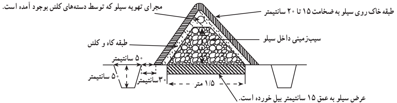
شکل ۲-۵- مقطع سیلوی سیب زمینی و محصولات مشابه
