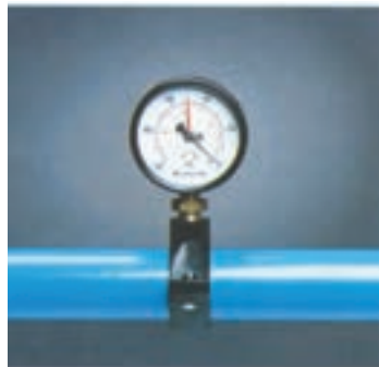
شکل ۳۹-۴- فشارسنج
