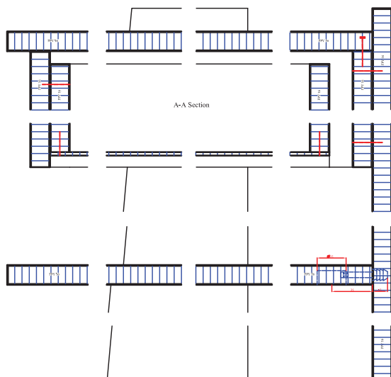
شکل ۸-۵ برش عمودی
