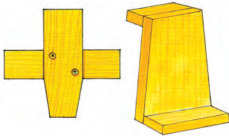
شکل ۴-۱-۱۰ شابلون اتصال دم چلچله
