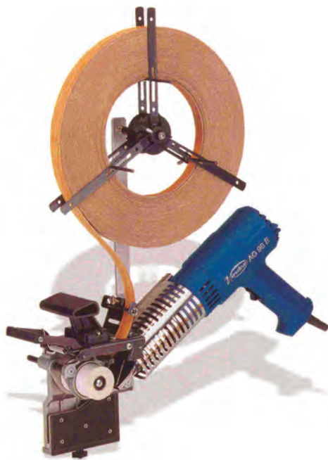
شکل ۶-۸۳ لبه چسبان برقی شسواری
