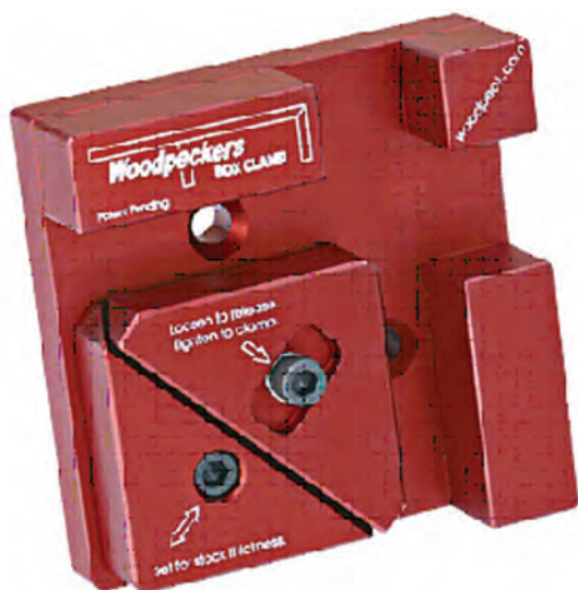
شکل ۳-۳۴ فیکسچر جهت مونتاژ قاب به حالت عمودی
