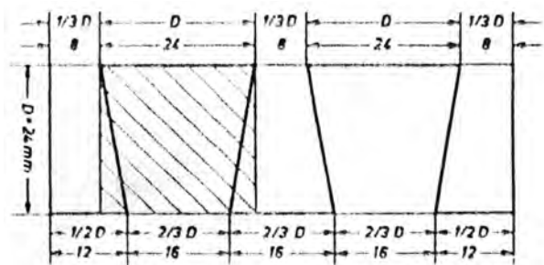
شکل ۴-۱-۱۰۲ نسبت‌های ترسیم شده اتصال دم چلچله ساده
