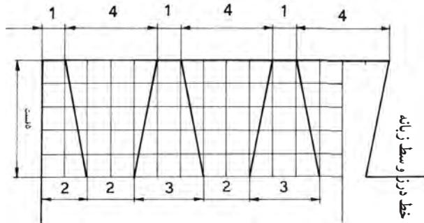
شکل ۴-۱-۱۰۴ روش ترسیم دم چلچله پنج‌قسمتی
