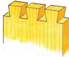
شکل ۴-۱-۱۰ اتصال دم چلچله ساده
