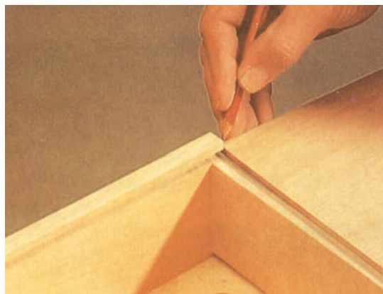
شکل ۱۵۸-۶ جاسازی کف کشو در جعبه کشو
