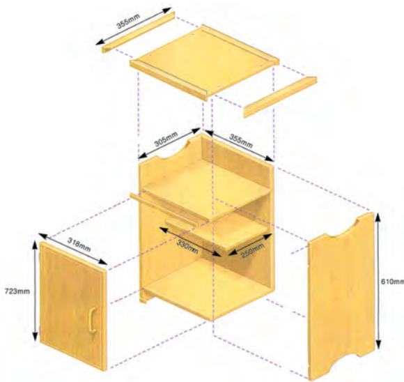
شکل ۸-۳۵ نقشه مونتاز قطعات کابینت
