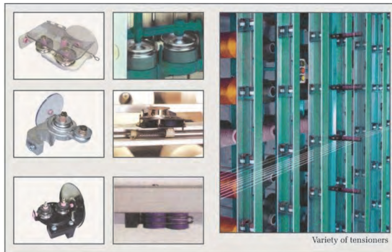
شکل ۹ انواع پولکی
