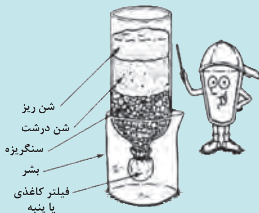
شکل ۵- صافی سازی آب
