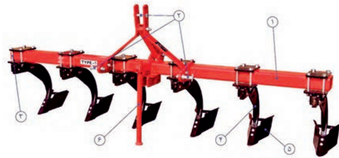
شکل ۱۳- ساختمان شیارکش
