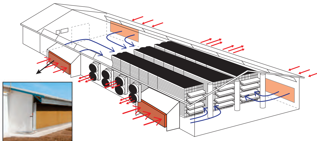
تهویه تونلی
