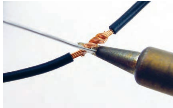
شکل ۴۵- لحیم کاری
