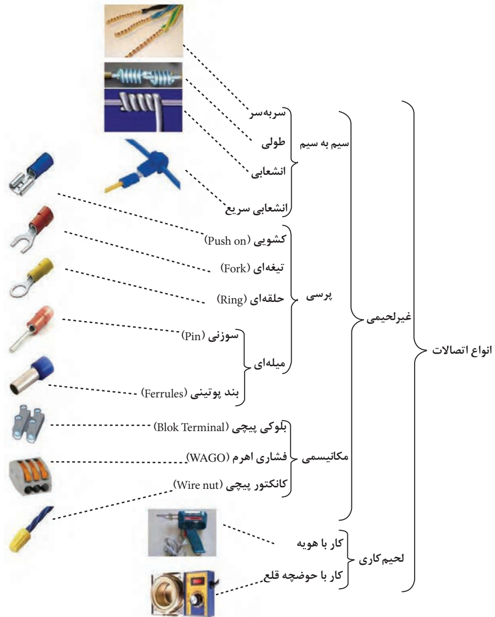
شکل ۲۰- انواع اتصالات
