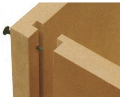
شکل ۲-۳۴- تصویر مجسم پشت بند دو راهه شده که داخل کنشکاف، با پیچ محکم می‌شود.
