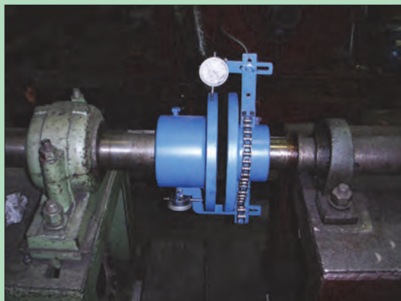
شکل ۷۷- هم‌راستا کردن محورها با ساعت اندازه‌گیری
