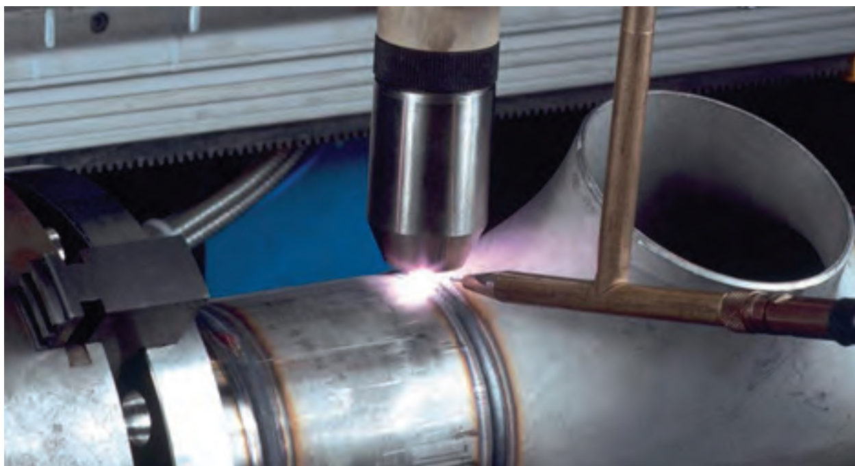
شکل ۲۸: جوشکاری قوس پلاسما
