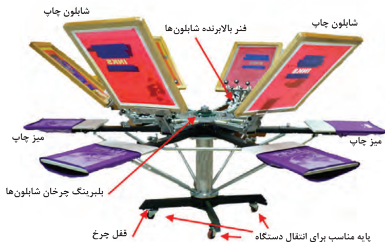
شکل ۱۹- دستگاه چاپ چند بازویی
