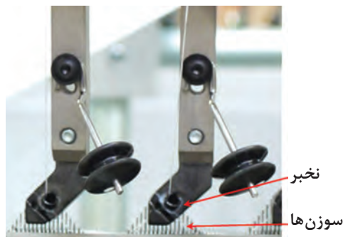
شکل ۳۰- تغذیه نخ به توسط نخبر
