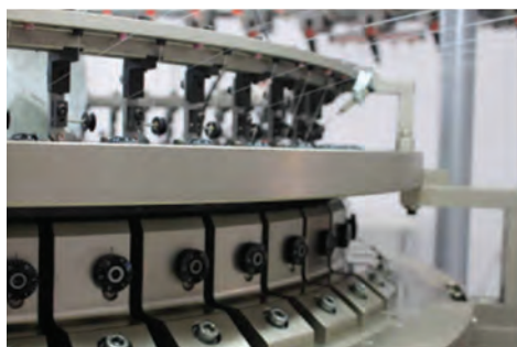
شکل ۳۴- سیلندر و اجزای روی آن در ماشین یک رو بافت
