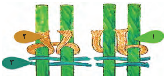
شکل ۲- گره فارسی گره ترکی
