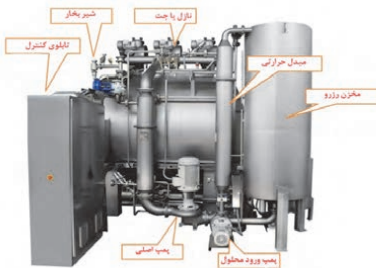
شکل ۷ تصویر قسمت‌های اصلی یک ماشین رنگری جت
