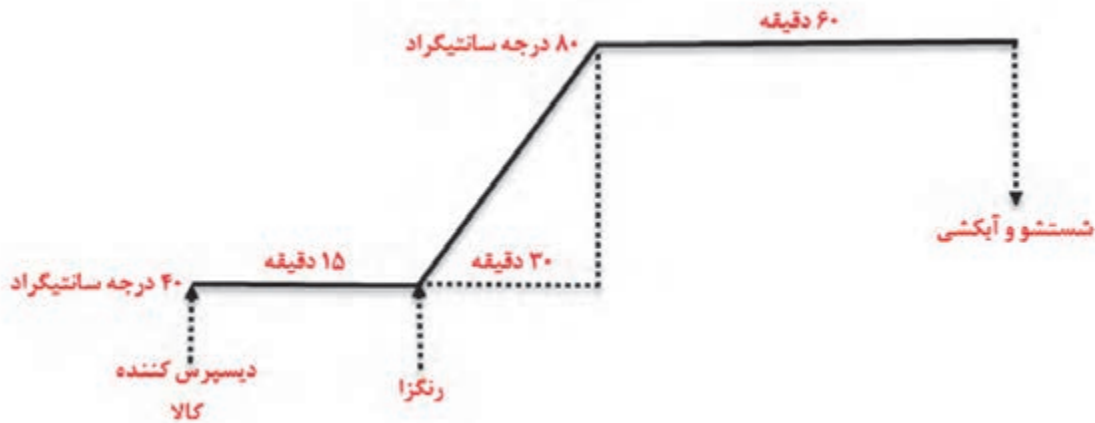
شکل ۱ تصویر نمودار رنگ‌رزی دی‌استات سلولز با مواد رنگ‌زای دیسپرس
