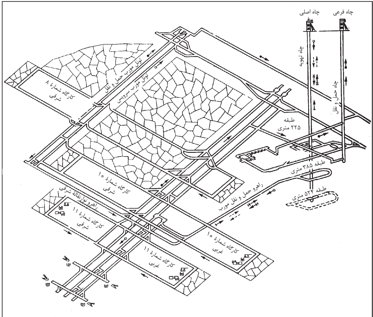
شکل ۱۱-۳- تهویه معدن
