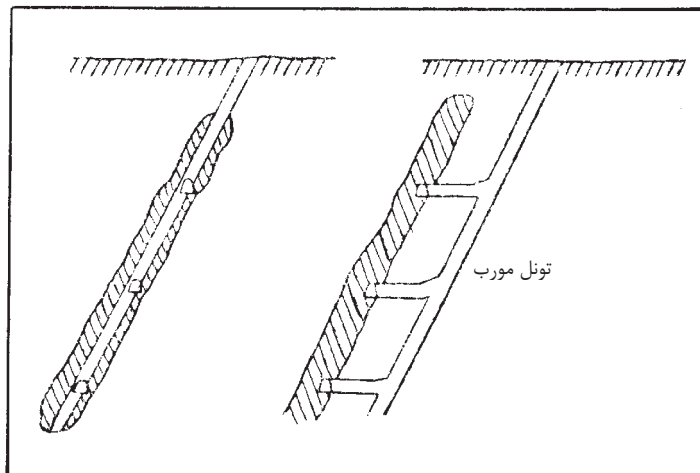
شکل ۲-۴- دسترسی به ماده معدنی توسط تونل مورب
