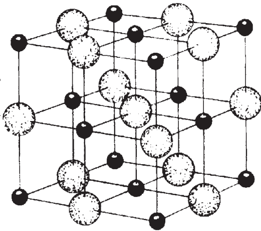
شکل ۲-۱۰- آرایش اتمی در سه جهت فضایی در بلور مکعبی نمک طعام
