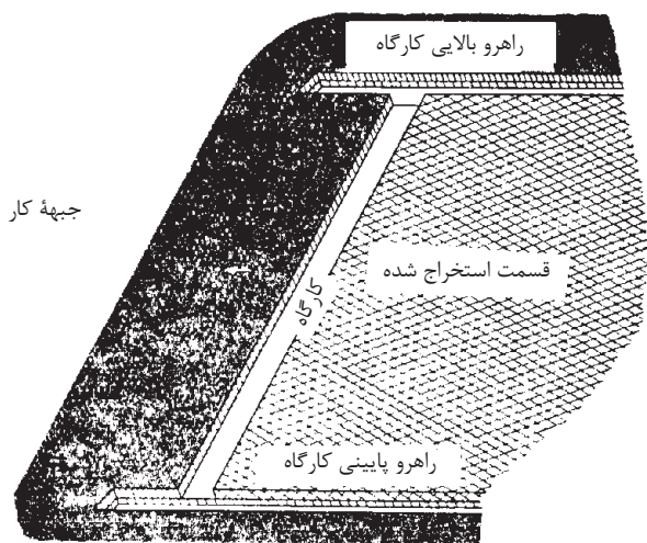
شکل ۳-۹- کارگاه استخراج
