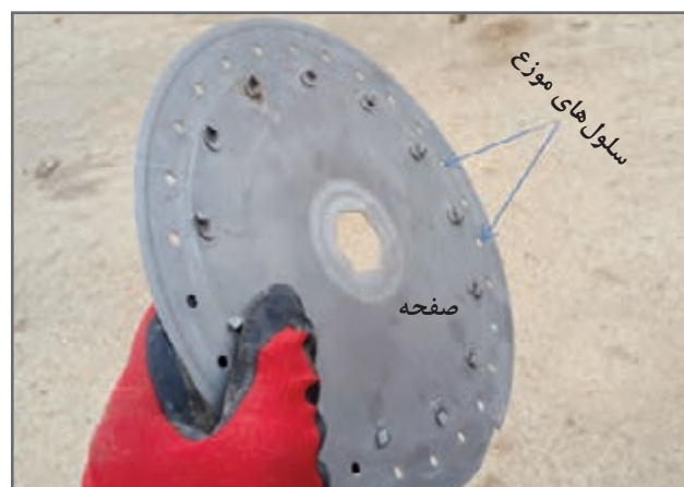
شکل ۲۳- دیسک صفحه موزع
