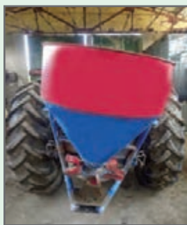
ب - تراز نبودن عرضی بذرپاش
