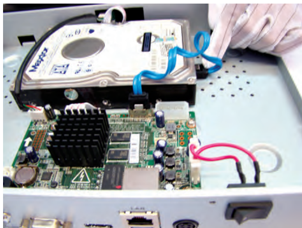
شکل ۳۳- اتصال کابل داده دیسک سخت
