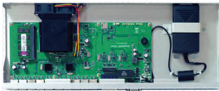
شکل ۴- نمای داخلی مسیریاب میکروتیک
