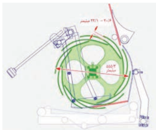
شکل ۴۶ - سایندر چهل پره
