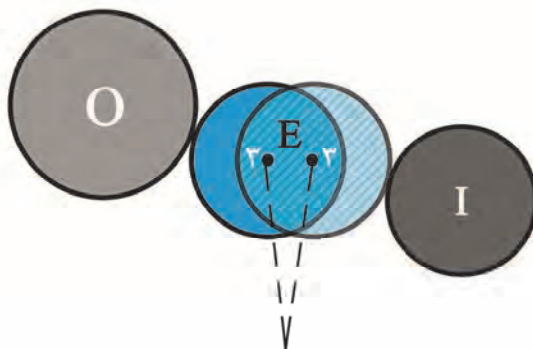
شکل ۲۰- فیلر کردن نورد رابط / داکتر
